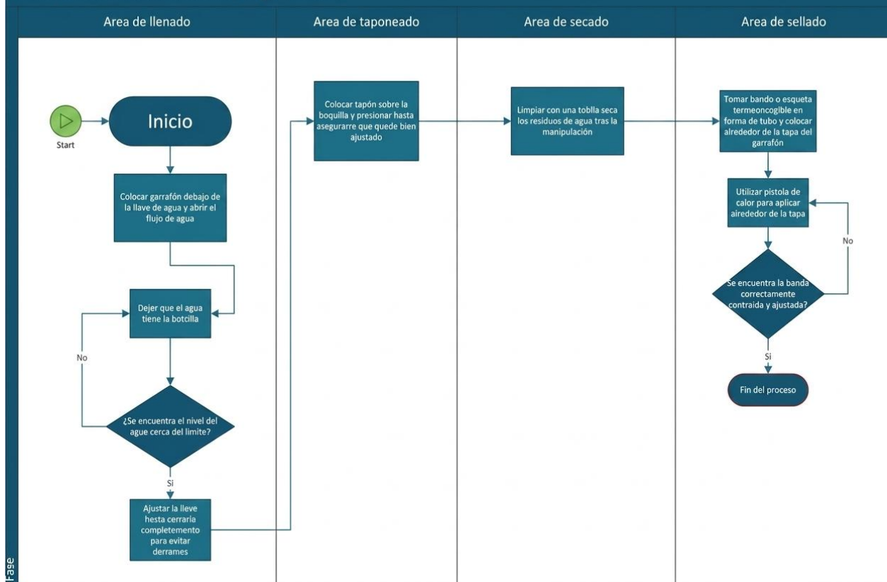
Proceso de acondicionamiento de garrafones
